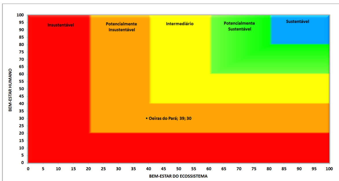
Figura 4 – Gráfico bidimensional do Barômetro da Sustentabilidade do município de Oeiras do Pará.
