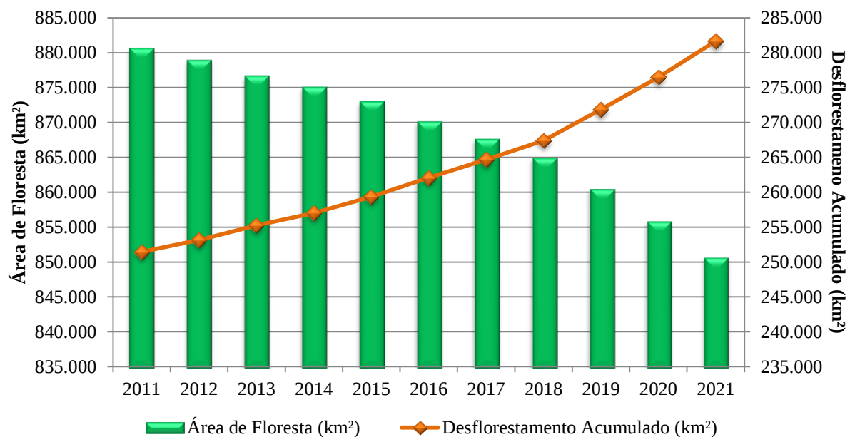
Gráfico 29. Área de Floresta (km²) e Desflorestamento Acumulado (km²) – 2010 a 2021.
