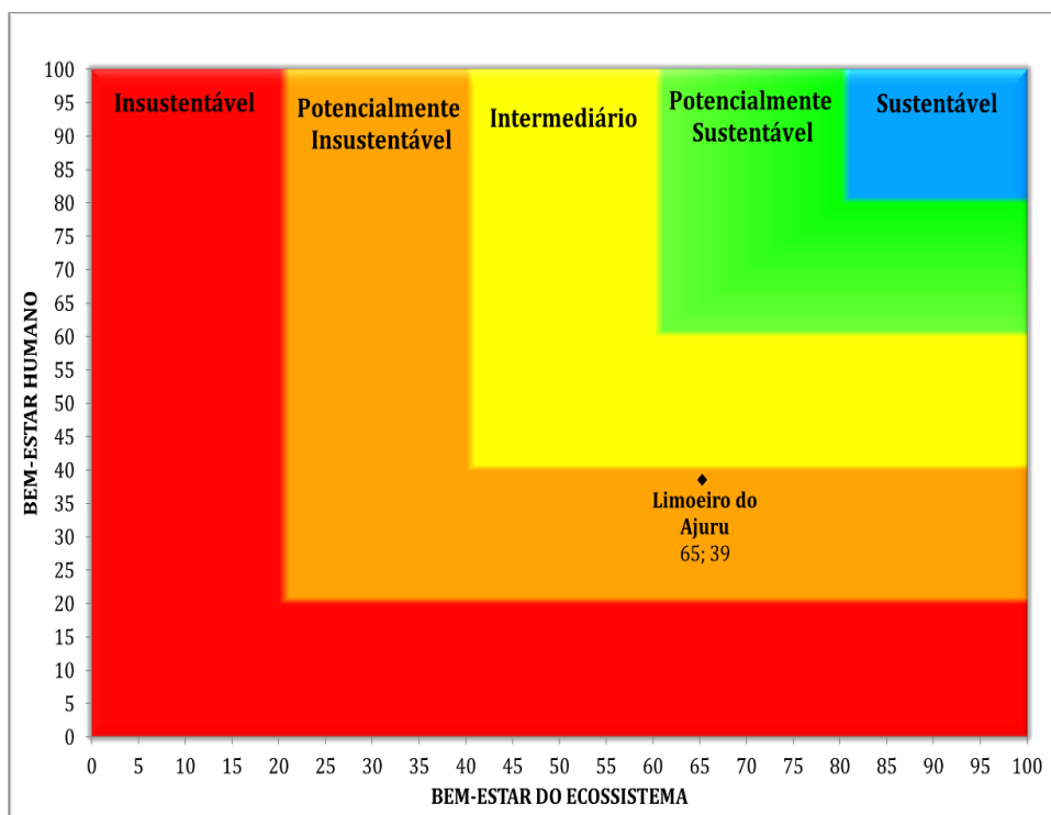
Figura 4 – Gráfico bidimensional do Barômetro da Sustentabilidade do município de Limoeiro do Ajuru
