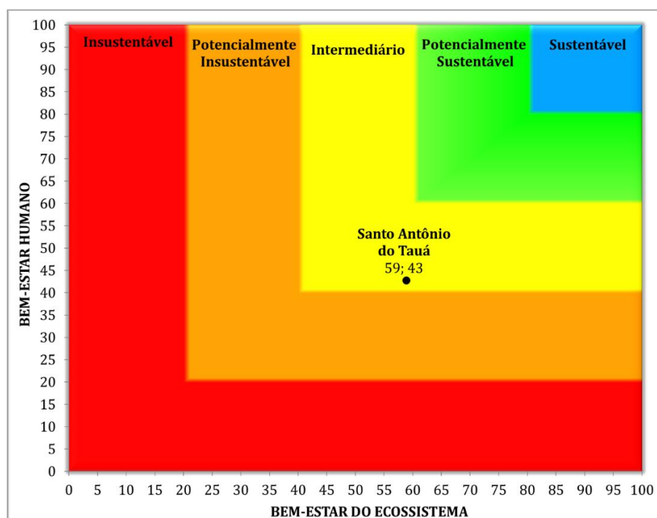
Figura 4 – Gráfico bidimensional do Barômetro da Sustentabilidade do município de Santo Antônio do Tauá
