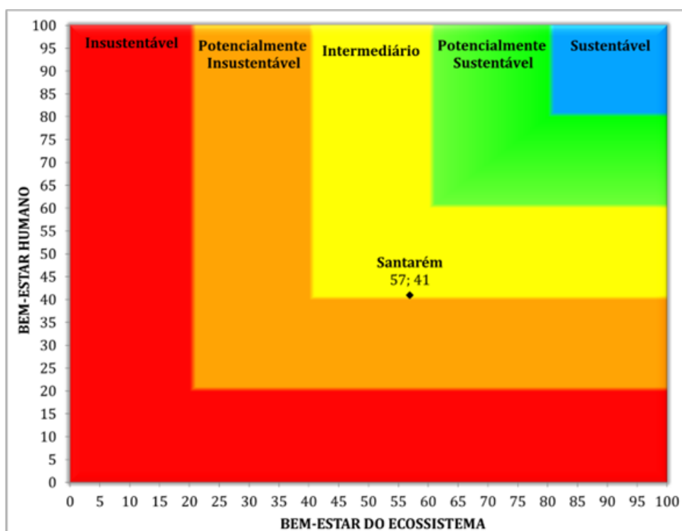
Figura 4 – Gráfico bidimensional do Barômetro da Sustentabilidade do município de Santarém
