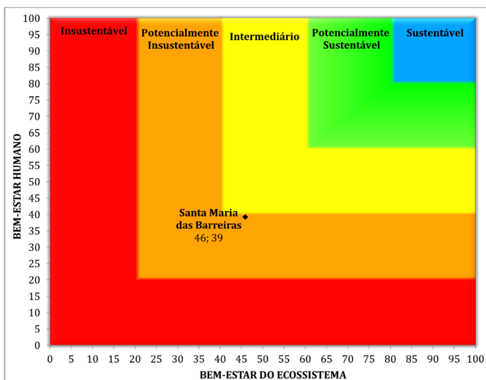
Figura 4 – Gráfico bidimensional do Barômetro da Sustentabilidade do município de Santa Maria das Barreiras
