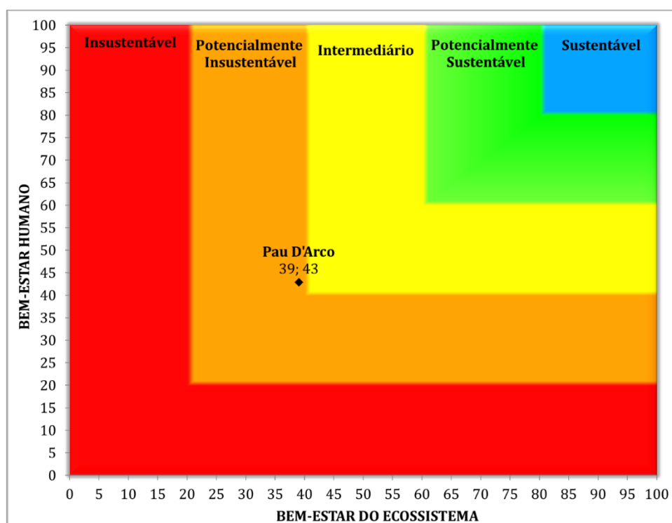
Figura 4 – Gráfico bidimensional do Barômetro da Sustentabilidade do município de Pau D’Arco
