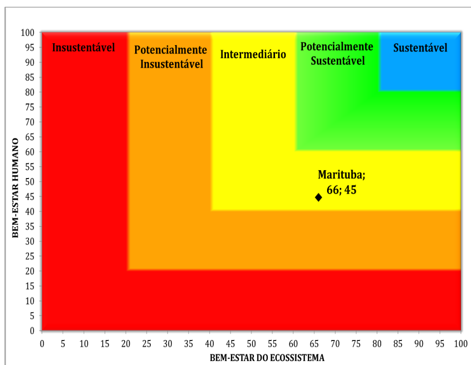
Figura 4 – Gráfico bidimensional do Barômetro da Sustentabilidade do município de Marituba
