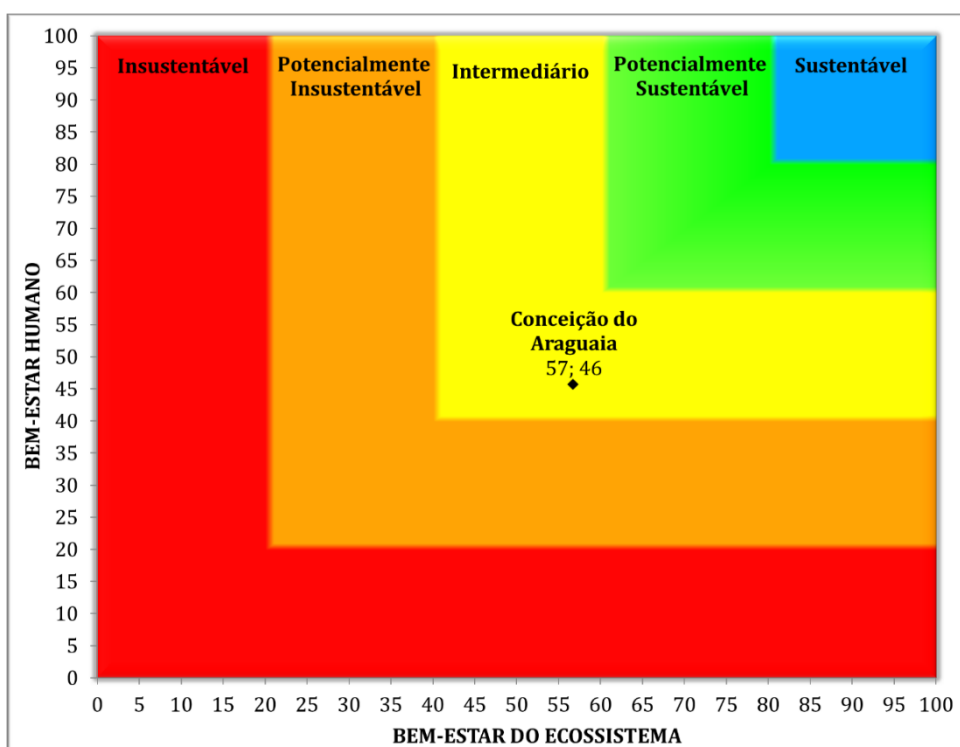
Figura 4 – Gráfico bidimensional do Barômetro da Sustentabilidade do município de Conceição do Araguaia
