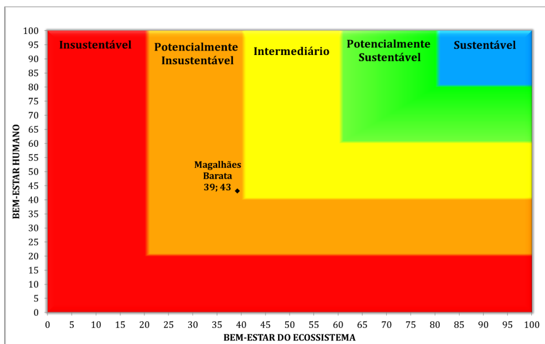
Figura 4 – Gráfico bidimensional do Barômetro da Sustentabilidade do município de Magalhães Barata
