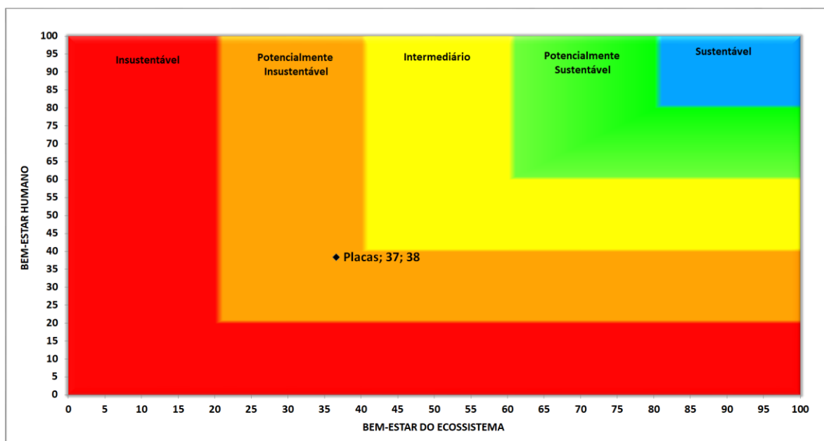
Figura 4 – Gráfico bidimensional do Barômetro da Sustentabilidade do município de Placas.
