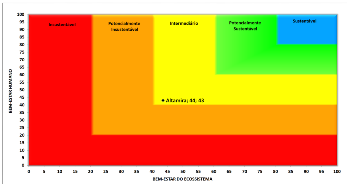
Figura 4 – Gráfico bidimensional do Barômetro da Sustentabilidade do município de Altamira.
